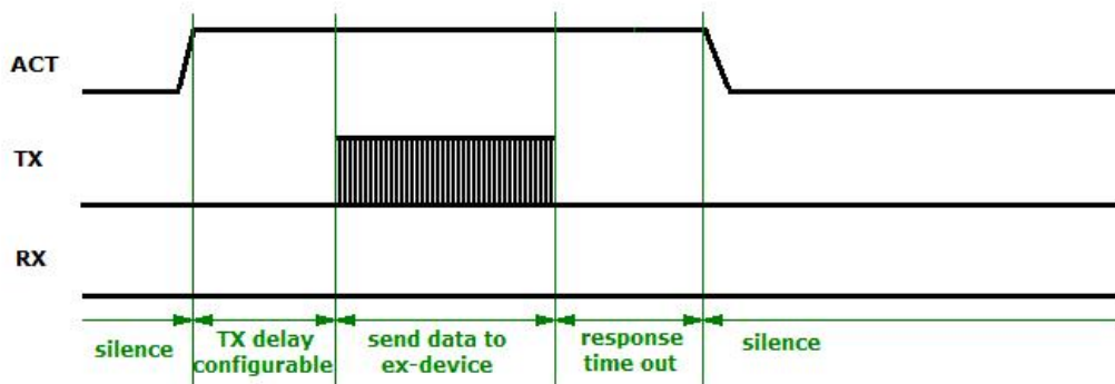
外设没有响应的 ACT、TX 和 RX 时序图
