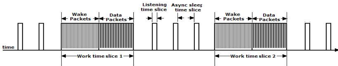
异步休眠示意图
